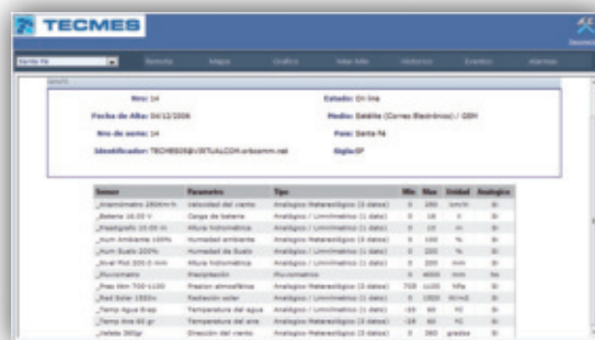
Datos de una estación remota seleccionada
