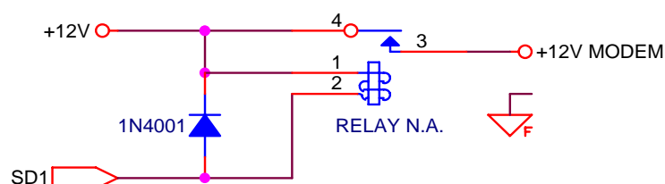
Circuito para conmutar la alimentación de los dispositivos de comunicación externos mediante la SD1
