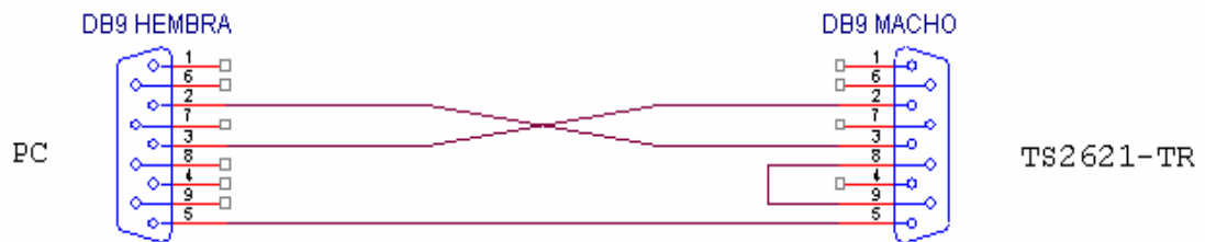
Cable de conexión entre PC y TS2621-TR
