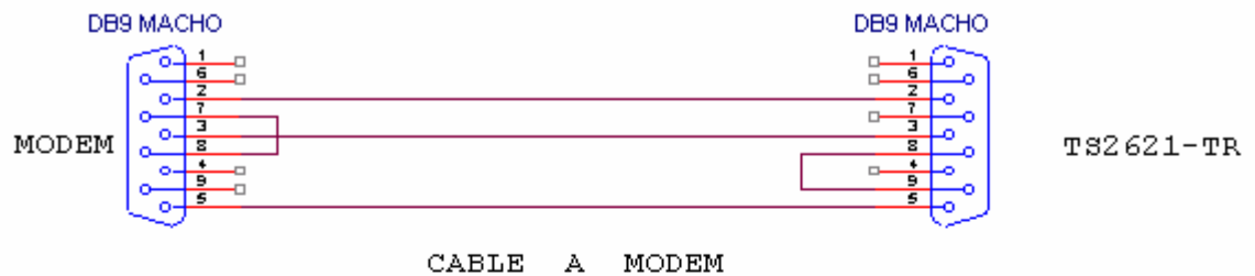
Cable de conexión entre Módem y TS2621-TR
